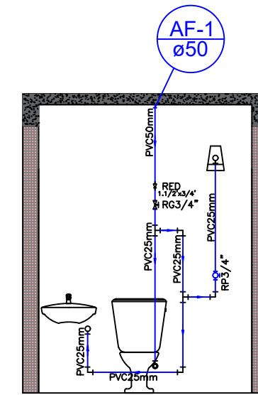
CORTE BB ESC. 1:50
