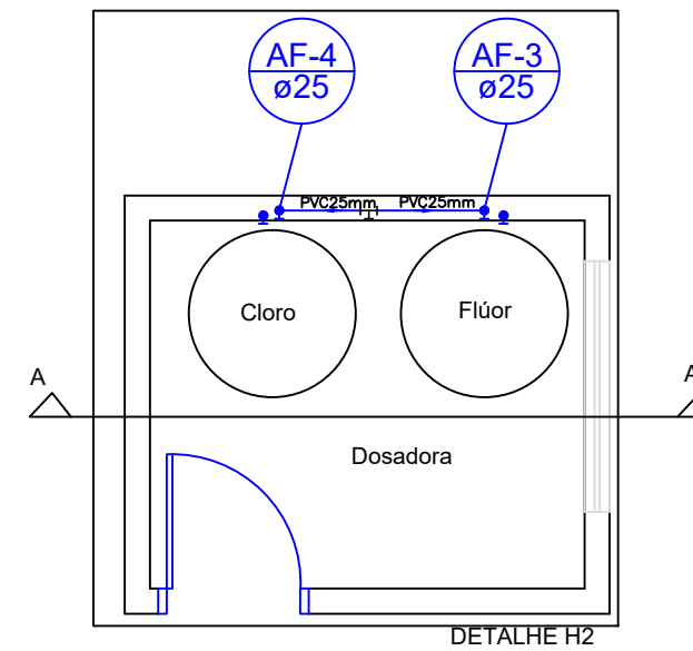
PROJETO HIDRÁULICA – PLANTA BAIXA ESC. 1:50
