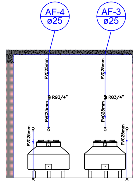
CORTE AA ESC. 1:50
