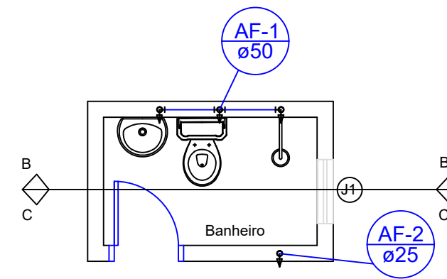
PROJETO HIDRÁULICA – PLANTA BAIXA ESC. 1:50
