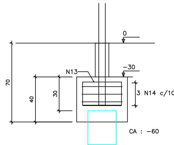
SEÇÃO TRANSVERSAL DO ARRANQUE, PILAR E VIGA BALDRAME ESC. 1:20
