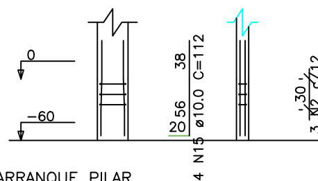
ARRANQUE PILAR ESC. 1:50
