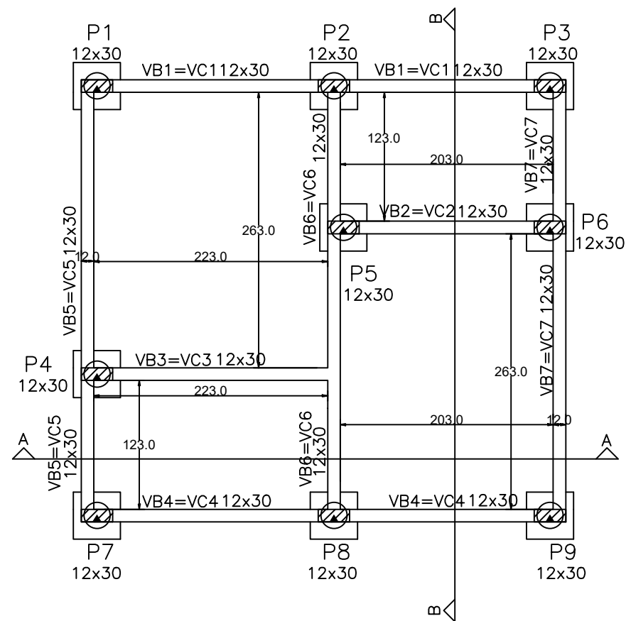
PROJETO ESTRUTURAL - PLANTA BAIXA ESC. 1:100
